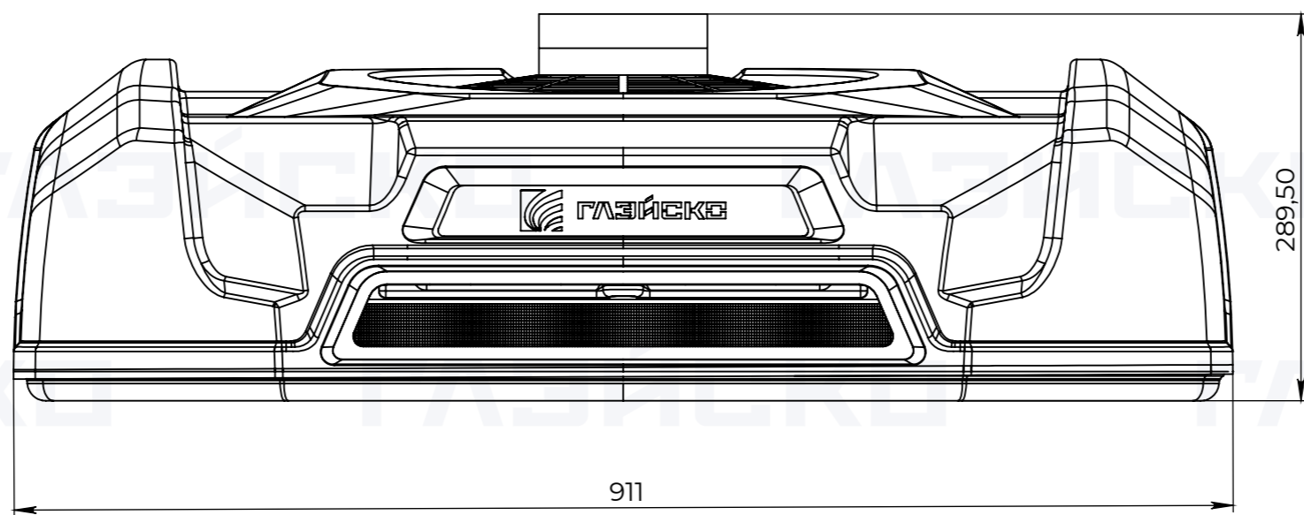
ВИД А МАСШТАБ 1:5
