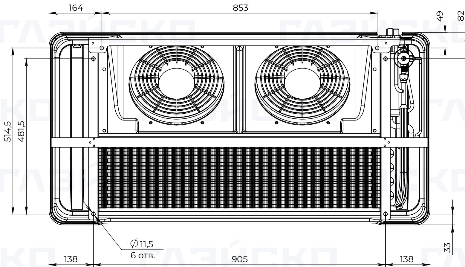
ВИД А (1:7)
